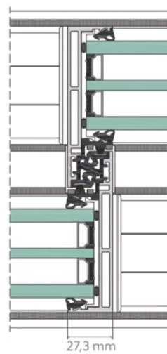
Querschnitt der Flügelverbindung
